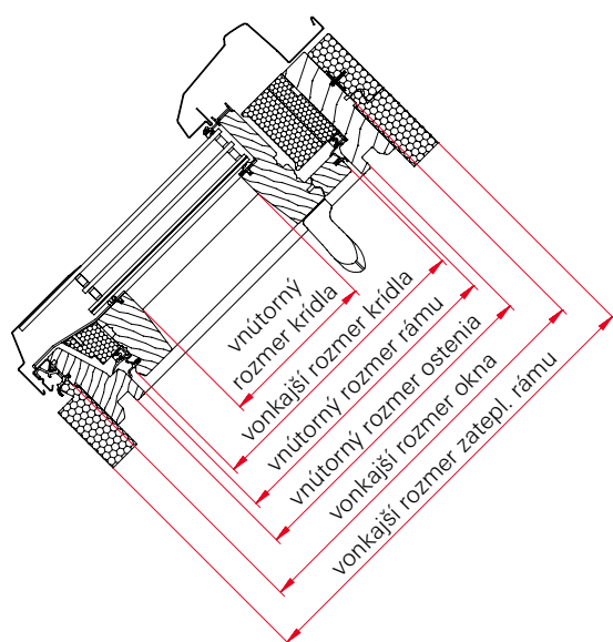
rez A-A
