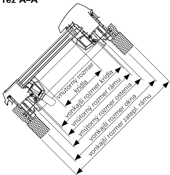
rez A-A
