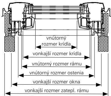
rez B–B
